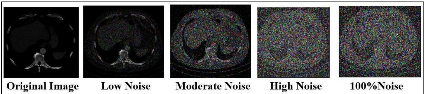
Fig 8: Forward Diffusion
