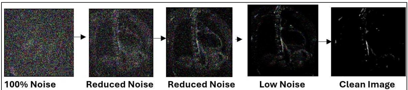
Fig 9: Reverse Diffusion
